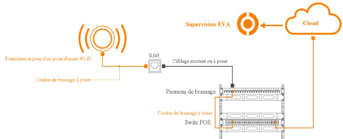
SCHEMA DE PRINCIPE D'INSTALLATION
